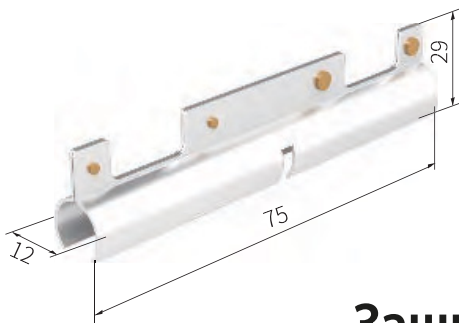
Характеристики стыковочного элемента с болтовым соединением
