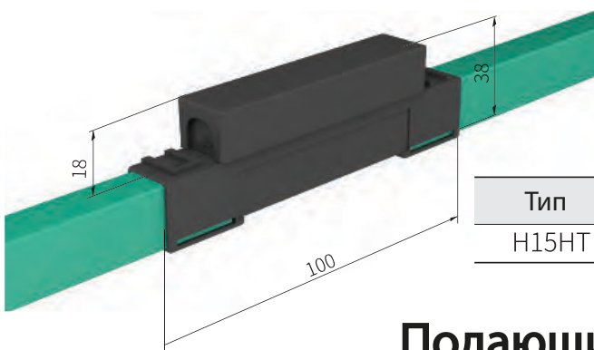
Характеристики защитного кожуха соединения
