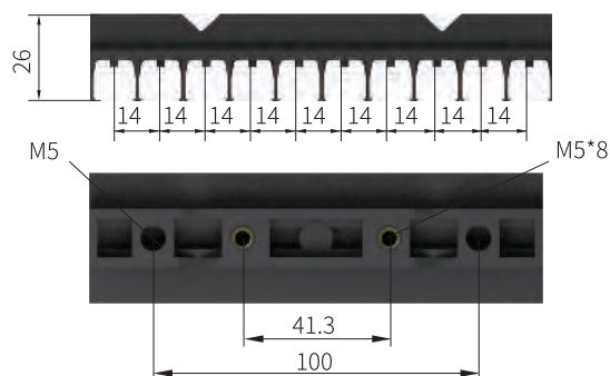
10-контактный подвес с болтами серии U1ZZJB10 Для I-образной балки
