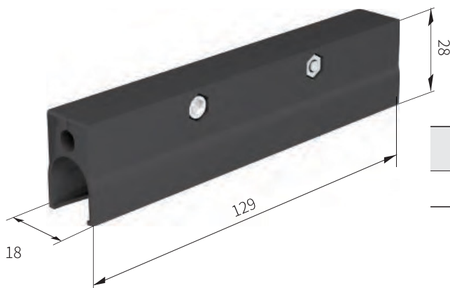
Характеристики защитного кожуха для стыков
