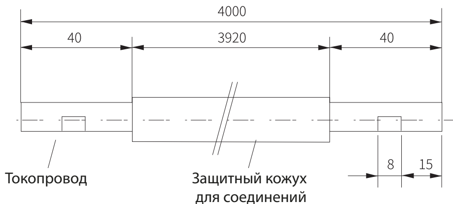
Характеристики шинопровода
