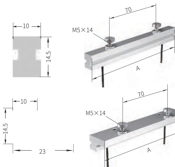
Характеристики крепежной панели для передающей направляющей
