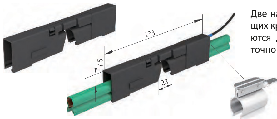
Характеристики изолирующего модуля
