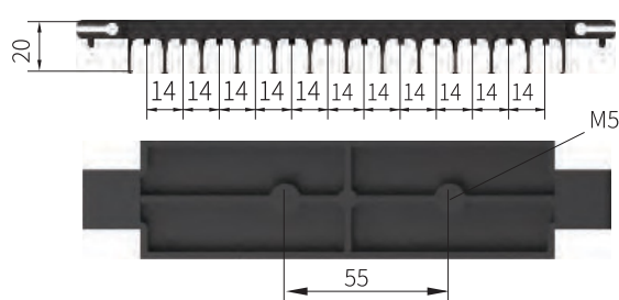
12-контактный защёлкивающийся подвес серии U1ZZJA12 (Алюминиевый трек ≈240 мм)
