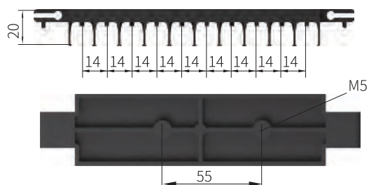
10-контактный защёлкивающийся подвес серии U1ZZJA10 (Алюминиевый трек ≈220 мм)
