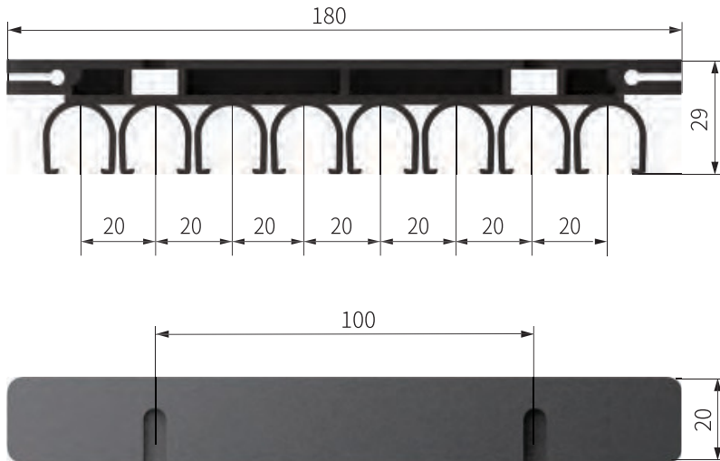
Характеристики 8-контактных кронштейнов
