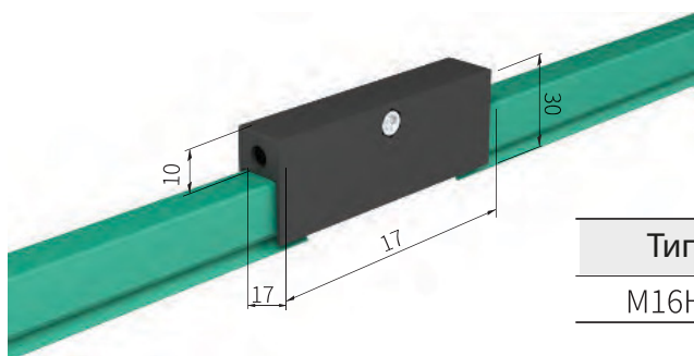
Характеристики защитного кожуха соединения
