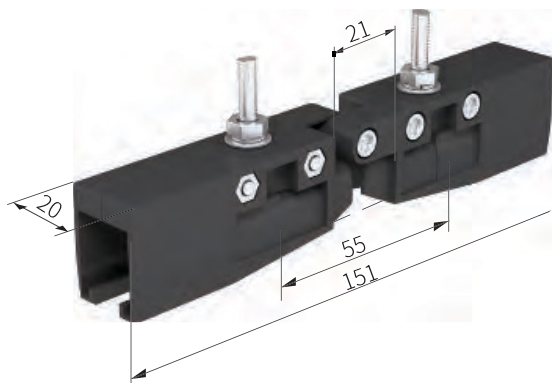
Характеристики изолирующего узла
