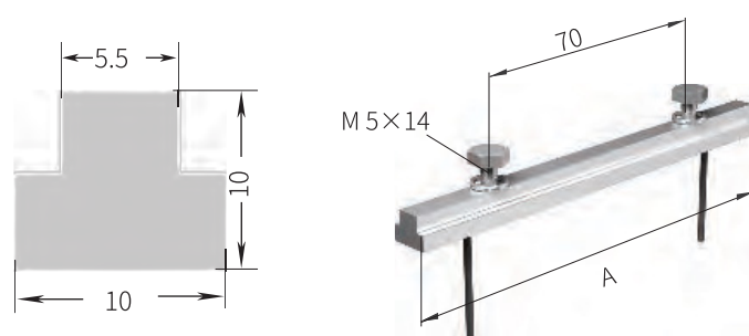
Характеристики крепежной панели для передающей направляющей
