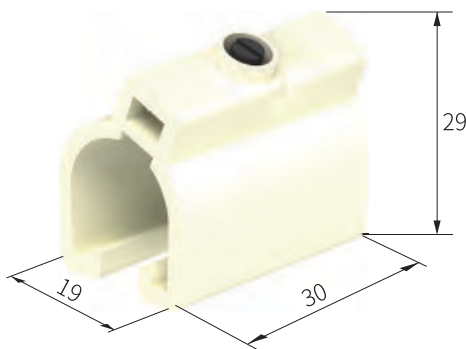
Характеристики защитного кожуха для клипсы подачи питания
